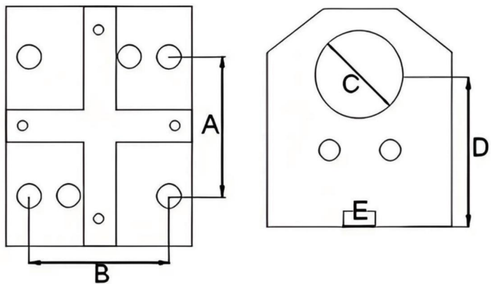
镗孔刀座参数表
